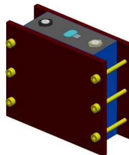
Fig. 4 Diagram of cell with clamp 图 4 电池上夹具图
